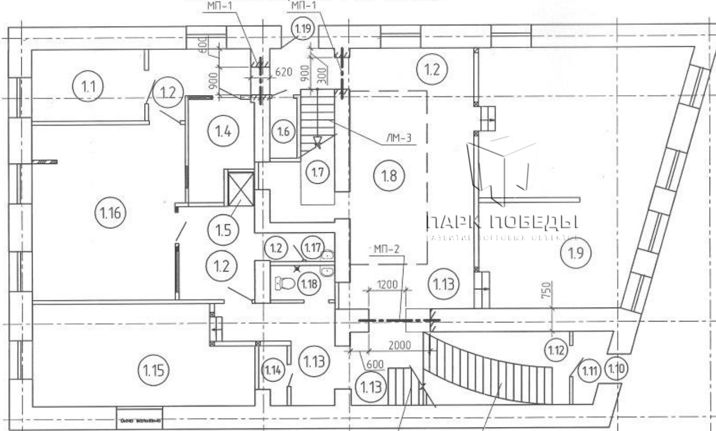
План помещений 1-го этажа
